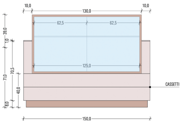
FIANCO
