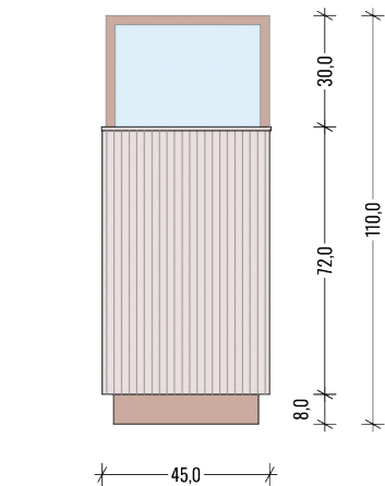
FIANCO
