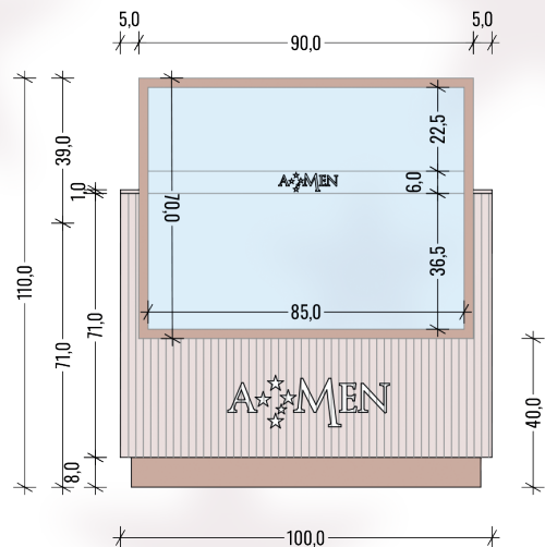
FRONTE
